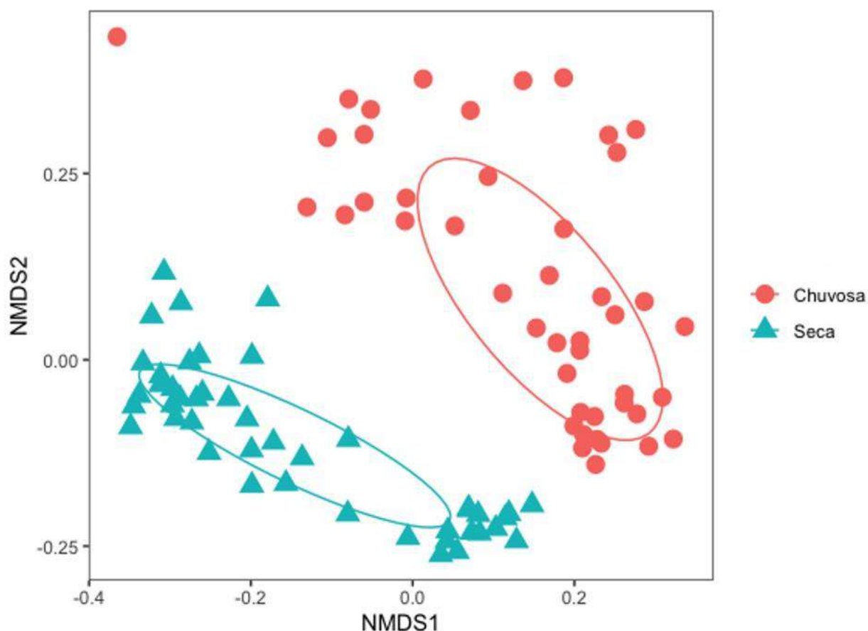
Figura 3 - Composição de espécies de fungos micorrízicos arbusculares (FMA) nas épocas seca e chuvosa na Ilha de Maracá. As elipses representam os agrupamentos dos FMA formados pela dissimilaridade da composição de espécies existente entre as estações. Cada ponto no gráfico representa uma amostra do solo em duas épocas de coleta.
