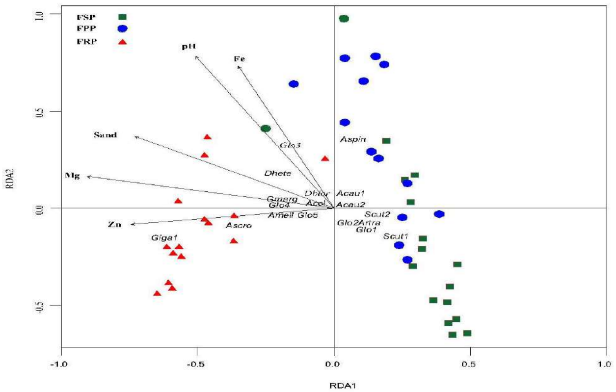
Figura 5 - Análise de Redundância (RDA) das comunidades de FMA com parâmetros de solo e tipos florestais na estação chuvosa da Ilha de Maracá, Brasil. Abreviação das espécies como na Tabela 4
