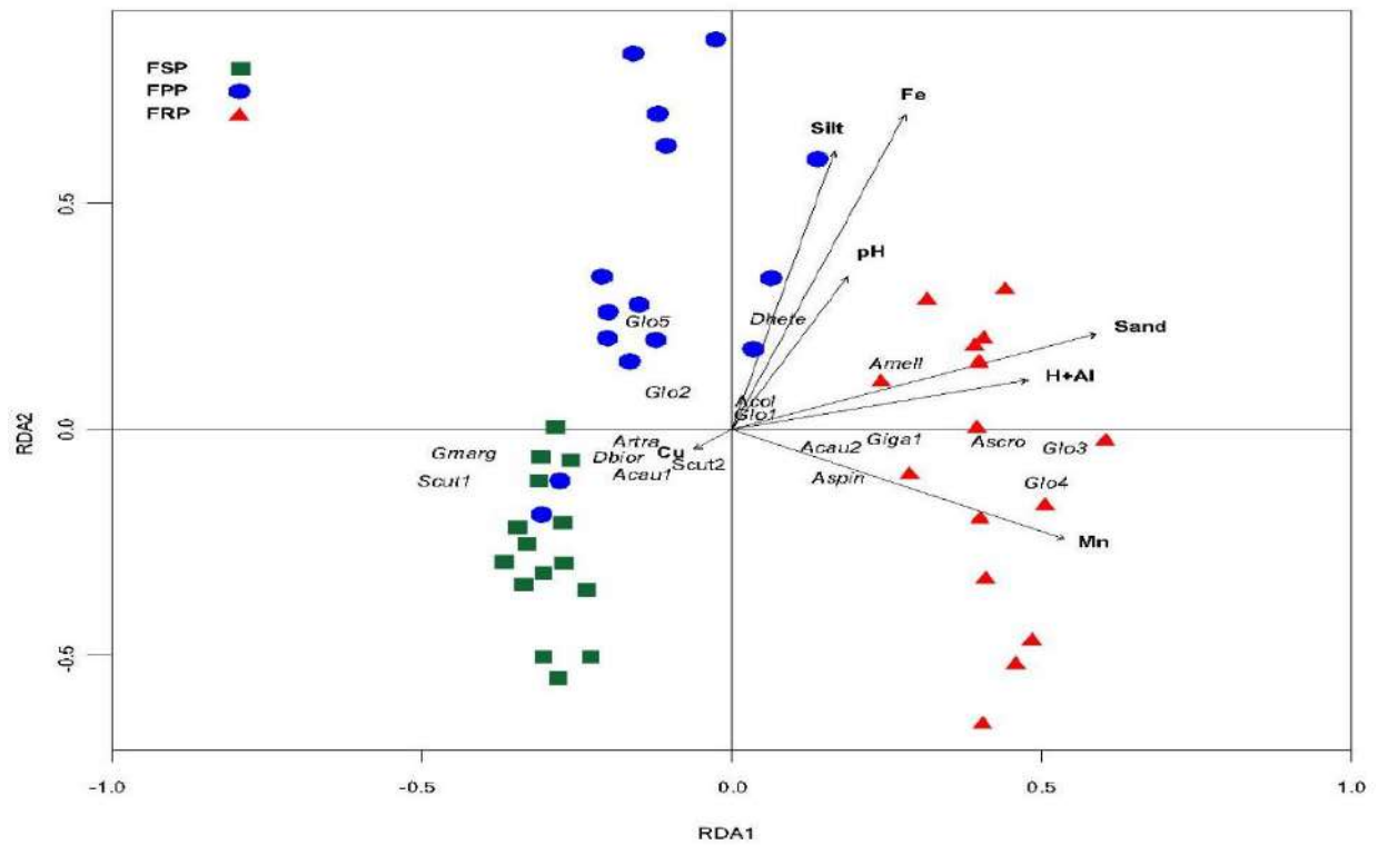
Figura 4 - Análise de Redundância (RDA) das comunidades de FMA com parâmetros de solo e tipos florestais na estação seca da Ilha de Maracá, Brasil. Abreviação das espécies como na Tabela 4.
