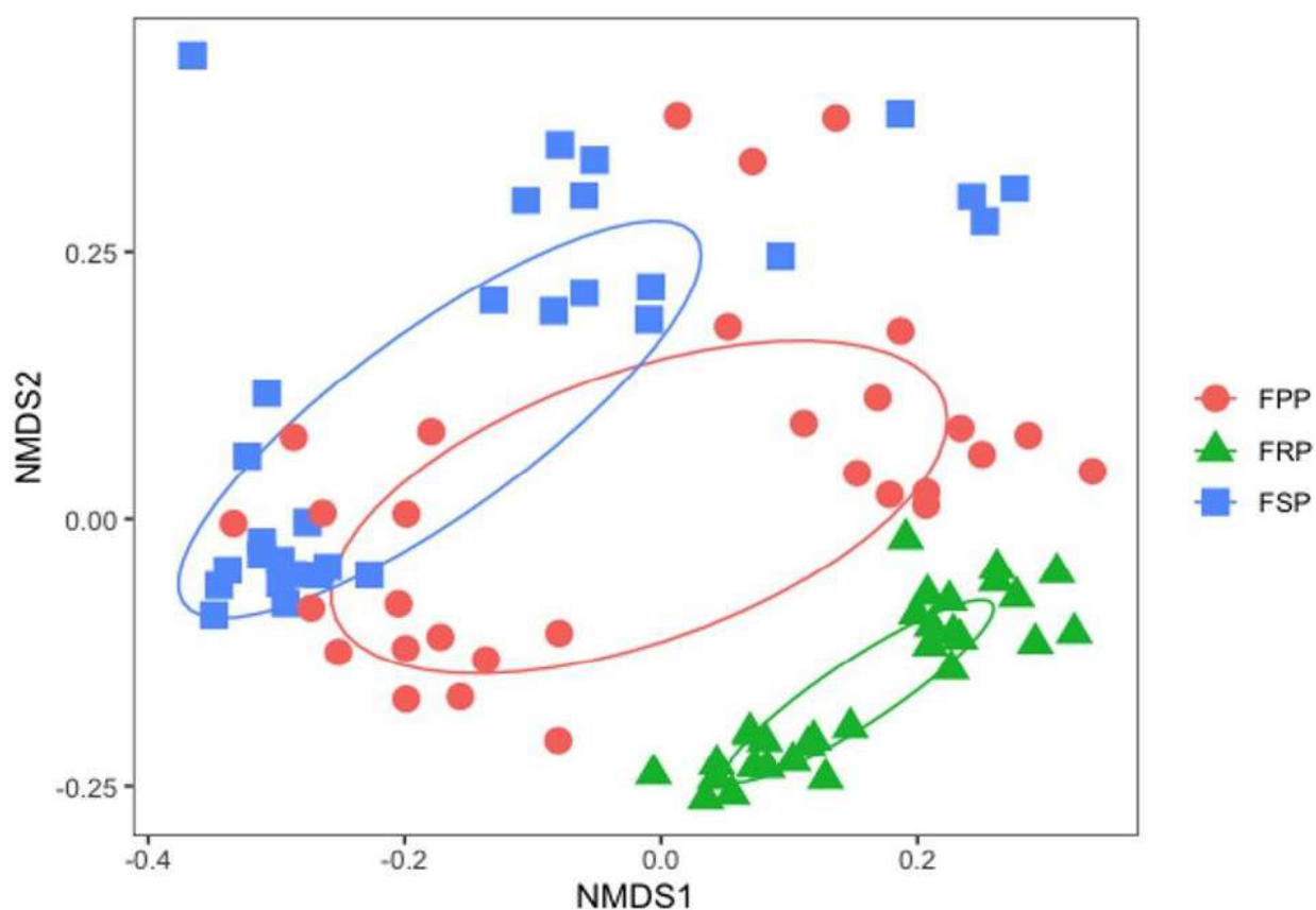
Figura 2 - Composição de espécies de fungos micorrízicos arbusculares (FMA) nos três tipos florestais (floresta sem Peltogyne , floresta pobre em Peltogyne e floresta rica em Peltogyne ) da Ilha de Maracá. As elipses representam os agrupamentos dos FMA formados pela dissimilaridade da composição de espécies existente entre as áreas. Cada ponto no gráfico representa uma amostra do solo em cada tipo de floresta nas duas épocas de coleta.
