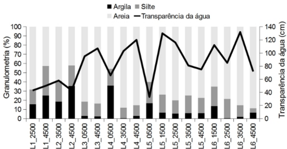
Fig. 1.10 Proporção de argila, silte e areia e a relação dos valores da transparência (mediana) nas parcelas aquáticas do Viruá. As parcelas encontram-se arranjadas ao longo do eixo das ordenadas pela sequência de trilhas.
