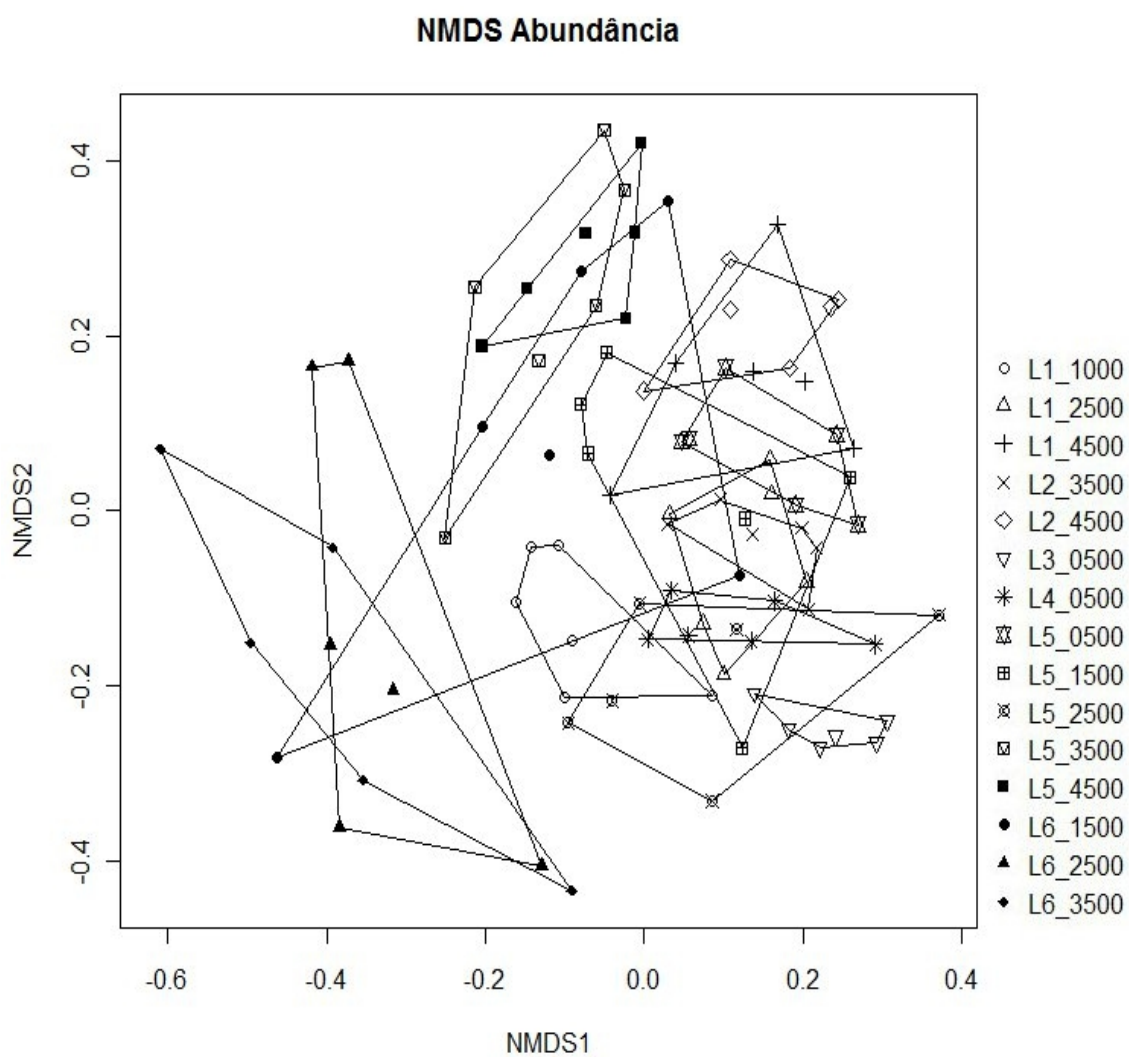
Fig. 2.6 - Ordenação por Escalonamento Multidimensional Não Métrico (NMDS) das parcelas aquáticas com base em dados de abundância das espécies de peixes em seis momentos de amostragem (início e final das chuvas, durante três anos consecutivos).
