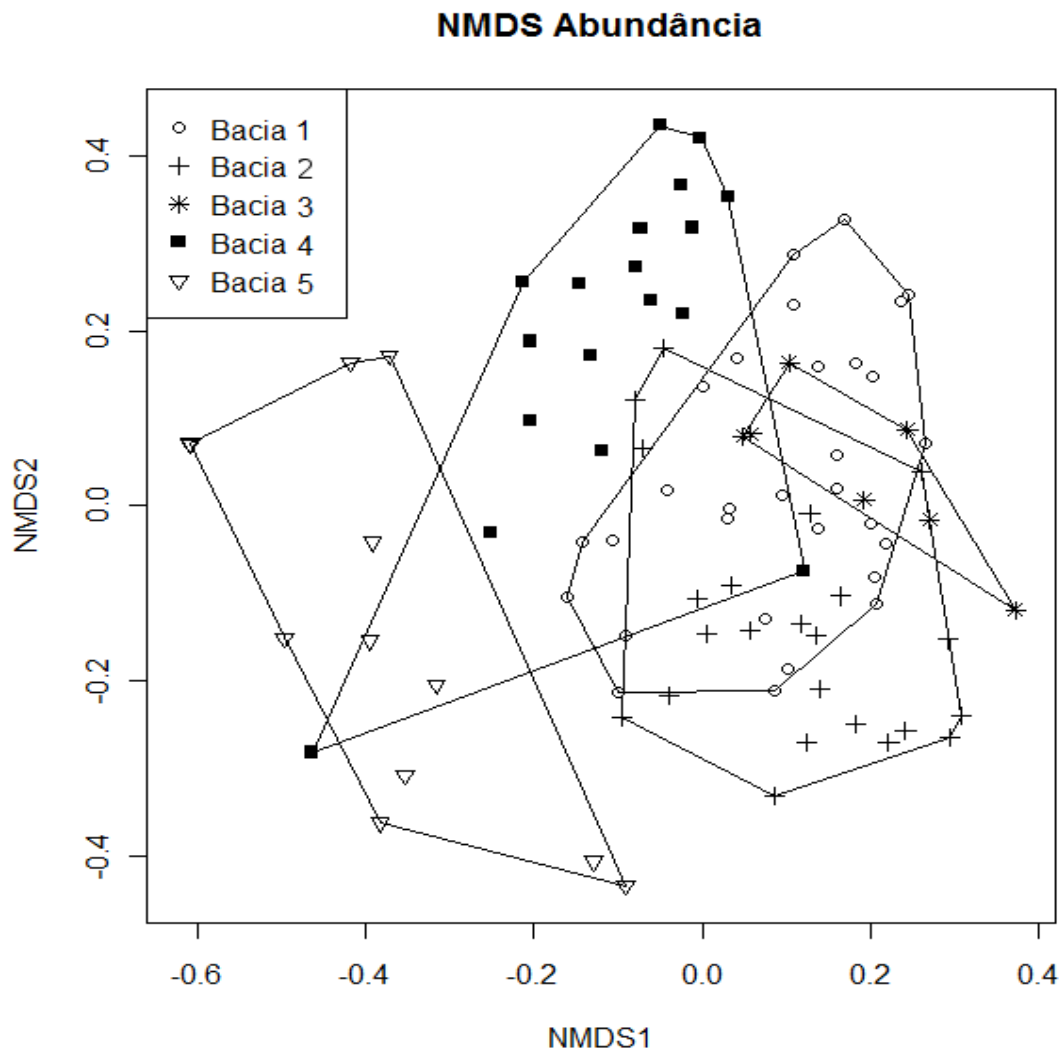
Fig. 2.11 - Ordenações por Escalonamento Multidimensional Não Métrico (NMDS) das parcelas aquáticas com base em dados de abundância das espécies de peixes em seis momentos de amostragem (início e final das chuvas, durante três anos consecutivos). Os símbolos representam os conjuntos de amostras de cada microbacia.
