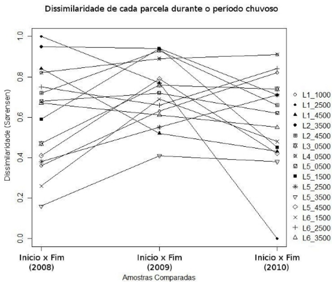
Fig. 2.5 – Valores de dissimilaridade (Sørensen) entre as assembleias do início e fim do período chuvoso de cada parcela.
