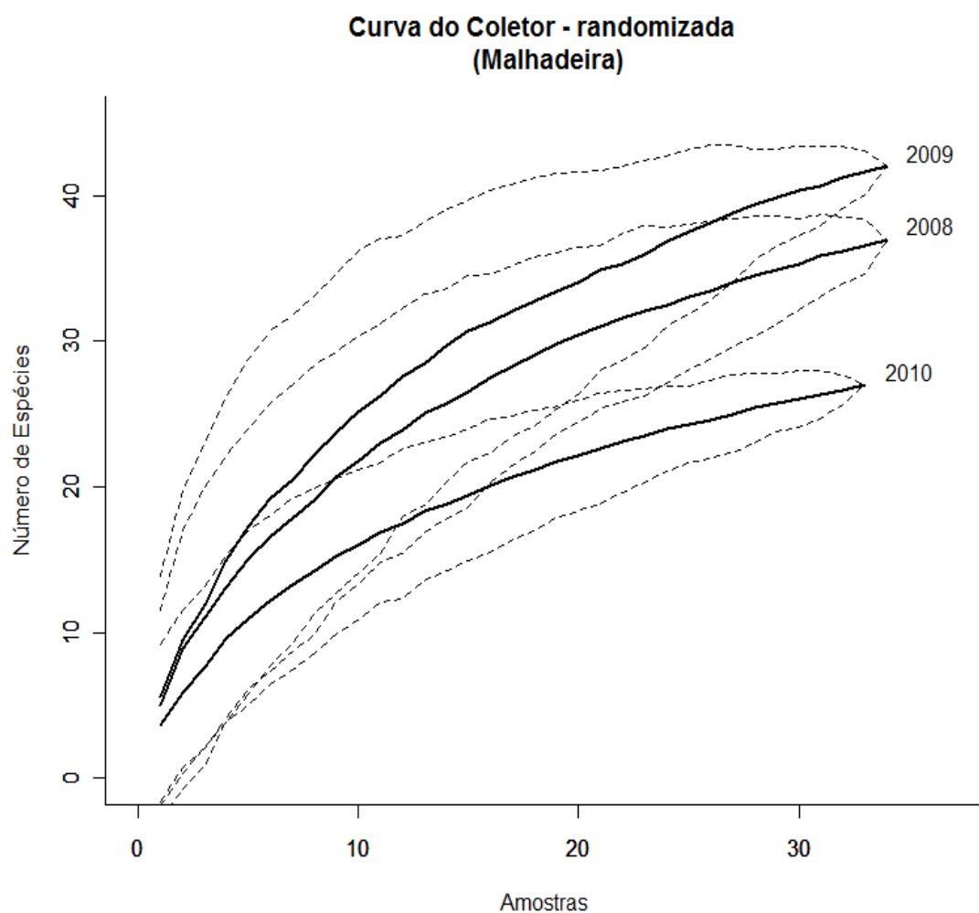
Fig. 2.4 – Curvas do coletor (randomizadas) e os intervalos de confiança (linhas pontilhadas) com base no número de parcelas amostradas com malhadeiras.
