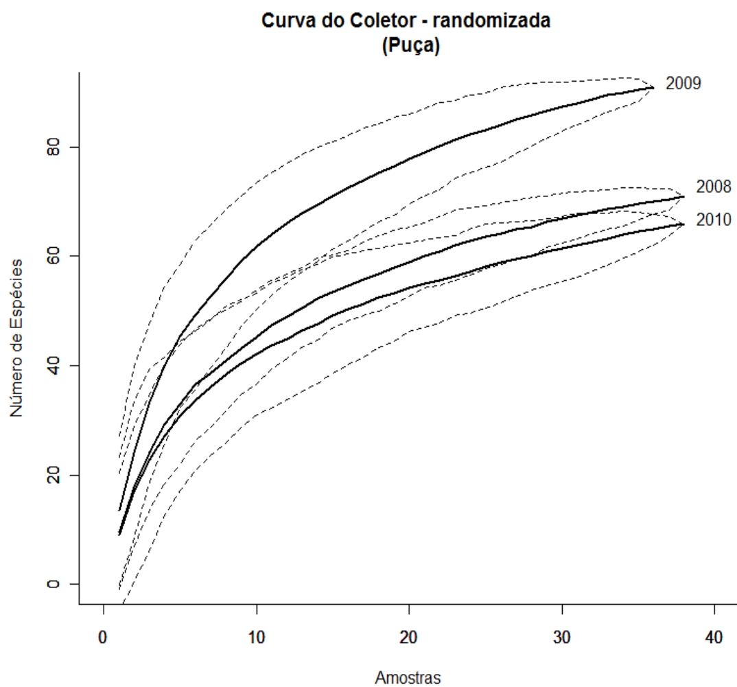
Fig. 2.3 – Curvas do coletor (randomizadas) e os intervalos de confiança (linhas pontilhadas) calculadas com base no número de parcelas para as amostras de peixes coletadas com puçá.
