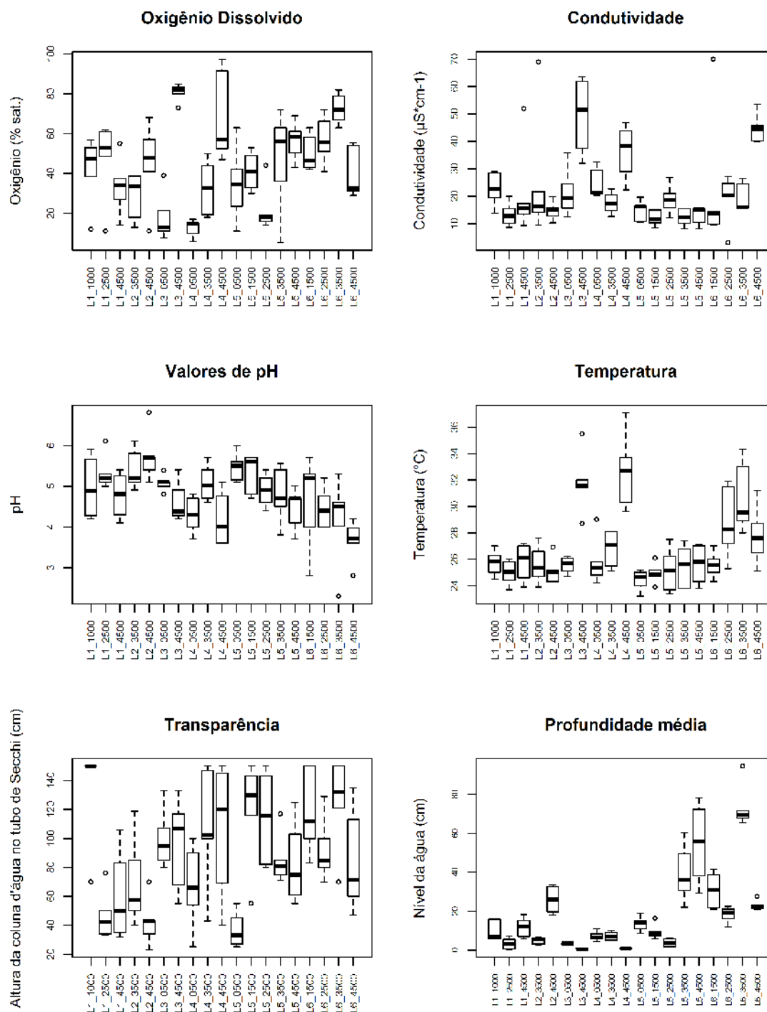
Fig. 1.4 Variáveis físicas e químicas das parcelas aquáticas do Viruá. Os círculos representam outliers , as linhas pontilhadas apresentam os quartis superior e/ou inferior +1,5\cdot\text{IQR} (amplitude interquartis) e a caixa representa os quartis superior e inferior em torno da mediana. As parcelas encontram-se arranjadas ao longo do eixo das ordenadas pela sequência de trilhas.
