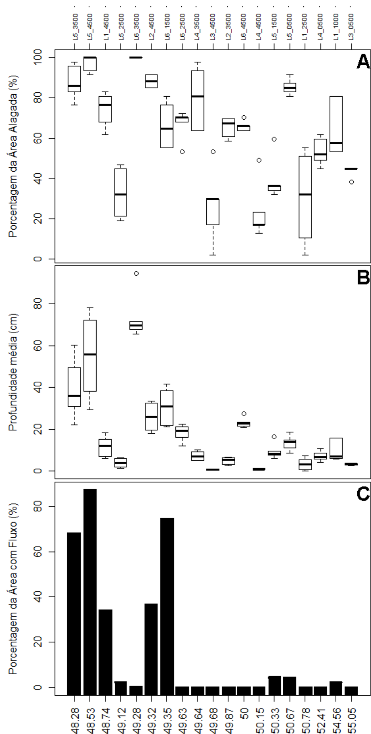
Fig. 1.6 Porcentagem da área alagada, profundidade média e porcentagem da área com fluxo superficial das parcelas aquáticas, ordenadas em função da altitude do terreno. Nas figuras A e B os círculos representam outliers , as linhas pontilhadas apresentam os quartis superiores e/ou inferiores +1,5 \cdot \text{IQR} (amplitude interquartil) e a caixa representa os quartis superior e inferior em torno da mediana, referentes às seis amostras que foram realizadas em cada parcela. Na figura C a medida foi feita em uma única amostragem.
