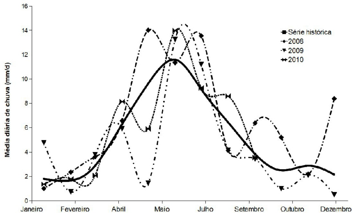
Fig. 1.2 Precipitação diária no município de Caracaraí – RR. A linha preta mais espessa representa a tendência de precipitação calculada com base na média mensal dos últimos 34 anos (1976 – 2010), as demais representam a precipitação dos três anos de amostra.
