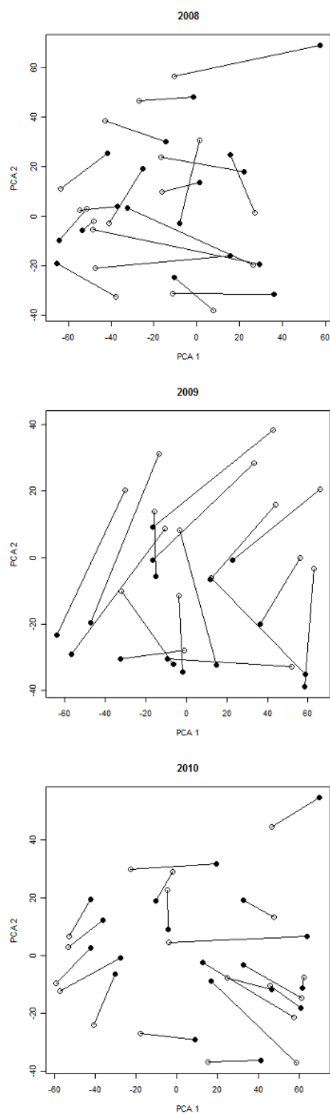
Fig. 1.9 Representação bidimensional da análise de ordenação (PCA) dos dados limnológicos nos três anos de amostragem (2008-2010), onde o círculo branco representa o início do período de chuvas, e o preto o final. O traço conecta as amostras de uma mesma parcela.
