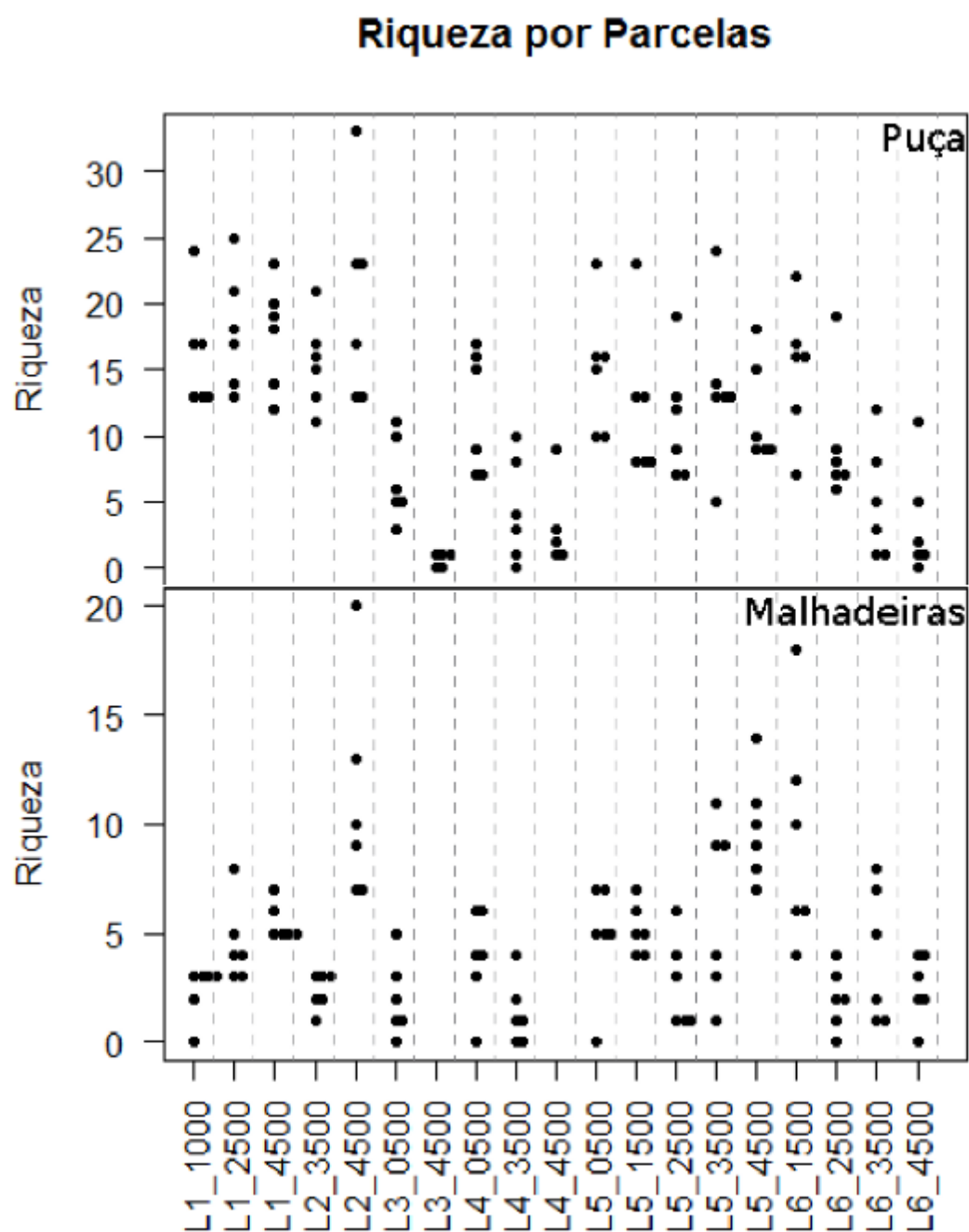
Fig. 2.2 – Riqueza de espécies por parcela para as coletas de puçá (acima) e malhadeiras (abaixo).
