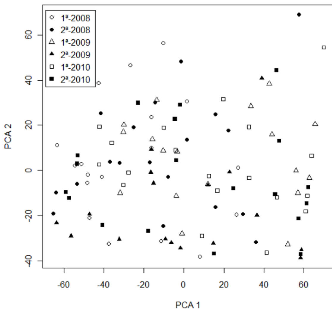
Fig 1.7 Representação bidimensional da análise de ordenação (PCA) das parcelas aquáticas em diferentes anos (2008-2010) entre o início e o fim do período chuvoso, com base nas características limnológicas.
