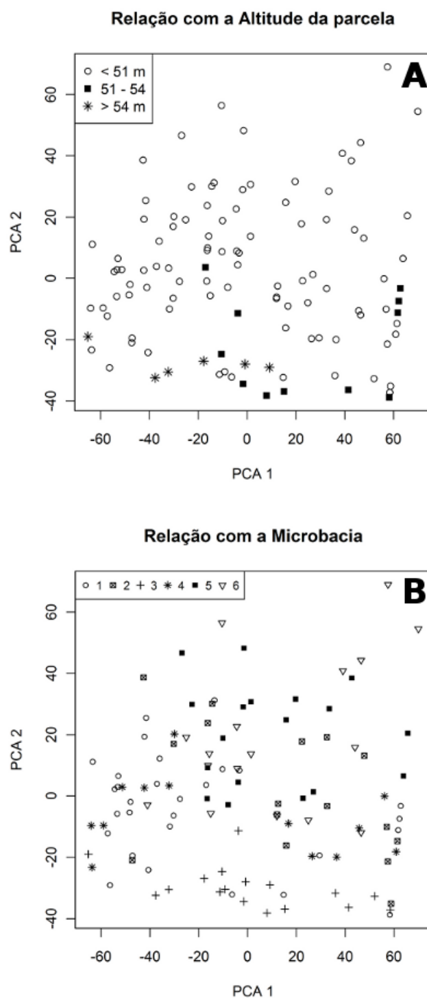
Fig. 1.8 Representação bidimensional da análise de ordenação (PCA) com as parcelas aquáticas de diferentes anos e início e fim do período chuvoso representados pelas três classes de altitude (A) e pelas microbacias (B).
