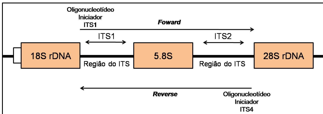
Figura 1 - Representação esquemática da região do rDNA com o espaço interno transcrito ITS1 e ITS2.
