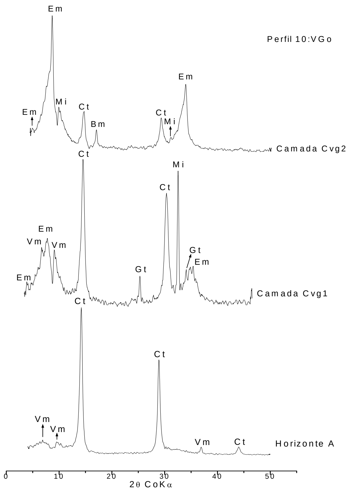
Figura 24 - Difrátogramas de raios-X da fração argila do VGo, perfil 10. Em-esmectita; Ct-caulinita; Vm-vermiculita; Gt-goethita; Bm-boemita; Mi-mica.
