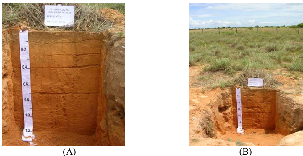
Figura 7 - Perfil 1, LAdx destacando a profundidade e coloração amarelada (A). Trincheira inserida na paisagem de relevo plano e vegetação do tipo savana graminosa (B).
