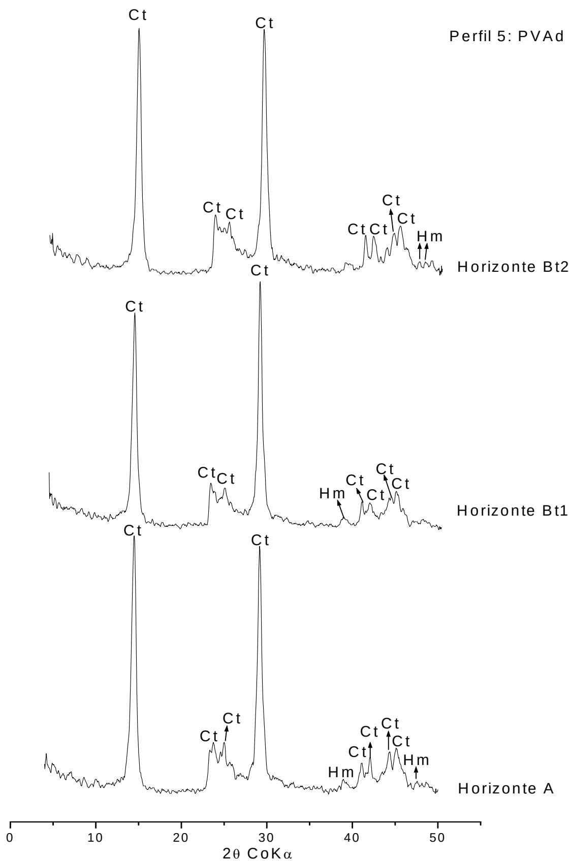
Figura 15 - Difractogramas de raios-X da fração argila do PVAd, perfil 5, horizontes A, Bt1 e Bt2. Ct-caulinita; Hm-hematita.
