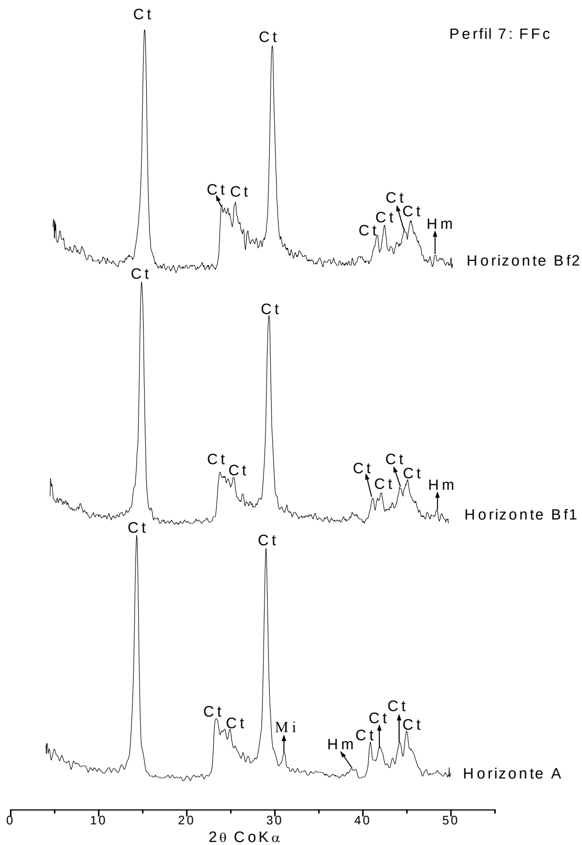
Figura 17 - Difratomogramas de raios-X da fração argila do FFc, perfil 7, horizontes A, Bf1 e Bf2. Ct-caulinita; Hm-hematita; Mi-mica.
