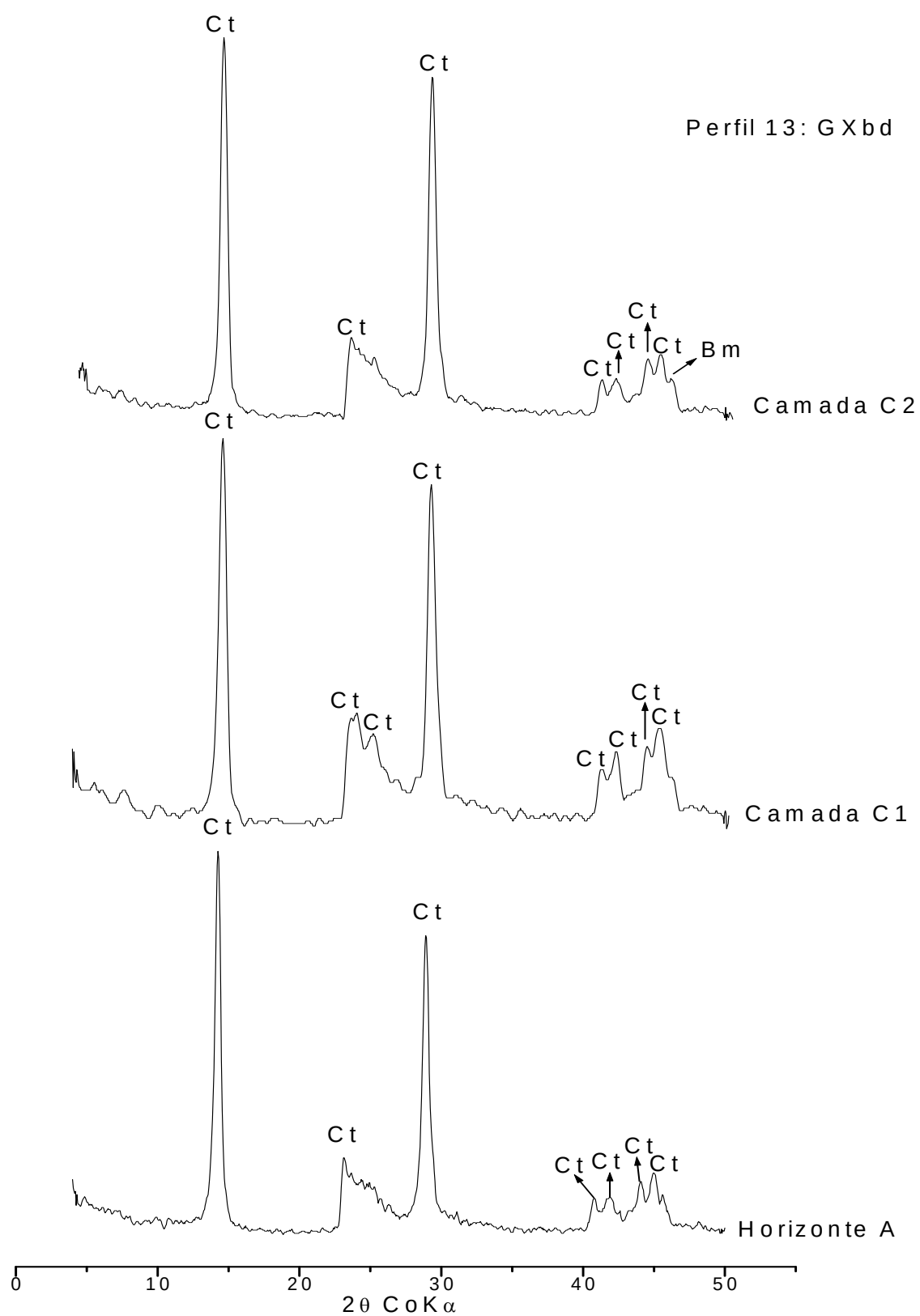
Figura 20 - Difrátogramas de raios-X da fração argila do GXbd, perfil 13, horizontes A, Bg1 e Bg2. Ct-caulinita; Bm-boemita.
