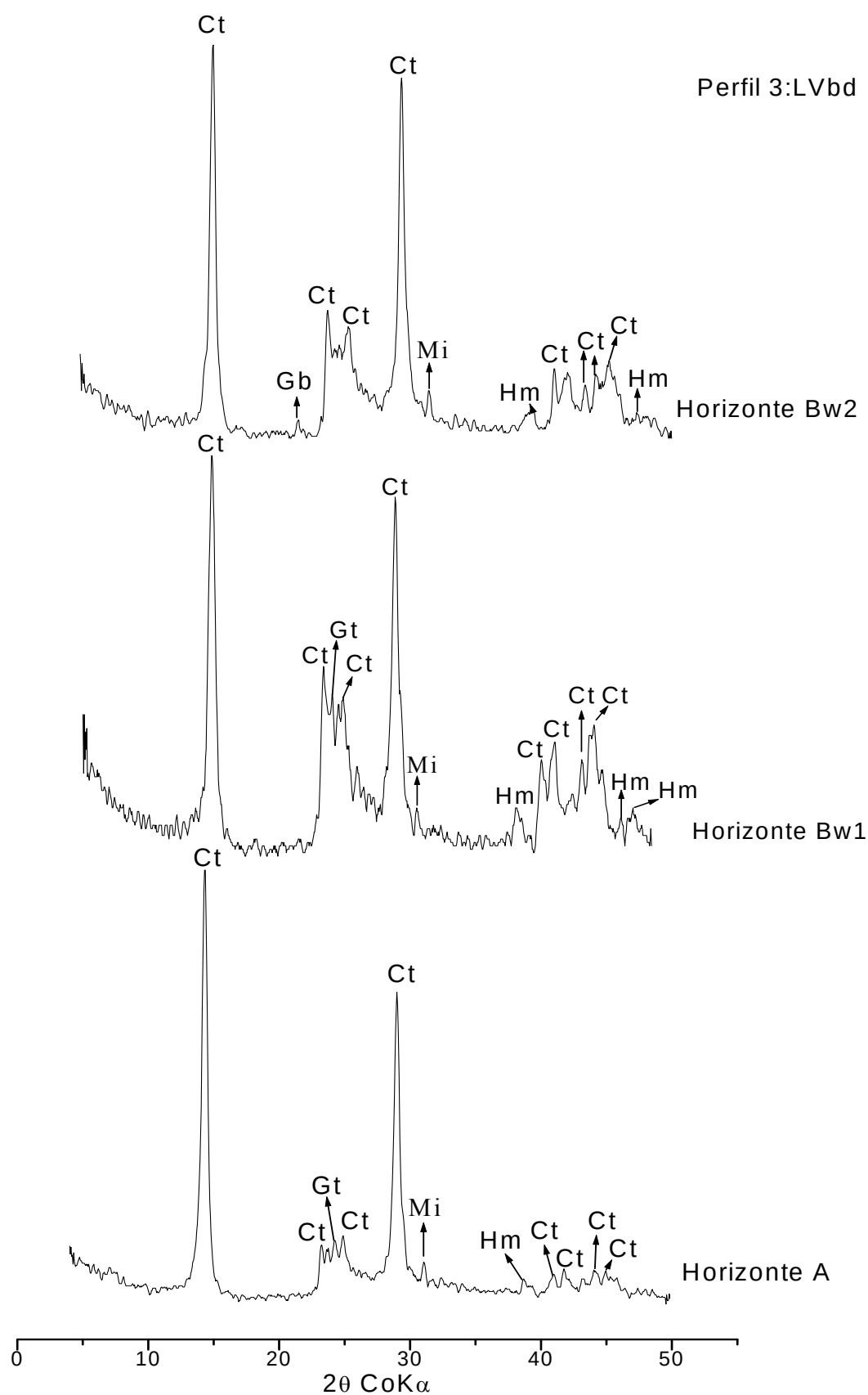
Figura 13 - Difrátogramas de raios-X da fração argila do LVd, perfil 3. Ct-caulinita; Hm-hematita; Mi-mica; Gt-goethita; Gb-gibsite.
