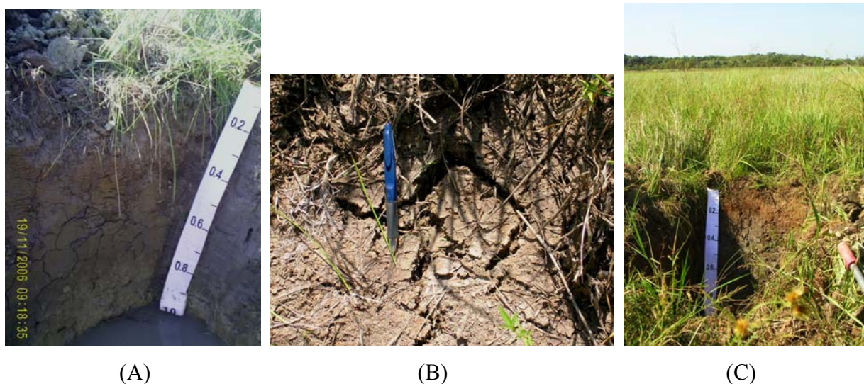
Figura 23 - Perfil de Vertissolo, mostrando o nível do lençol freático e fendilhamento (A), fendilhamento na superfície do solo (B) e a paisagem de domínio em relevo abaciado (C).
